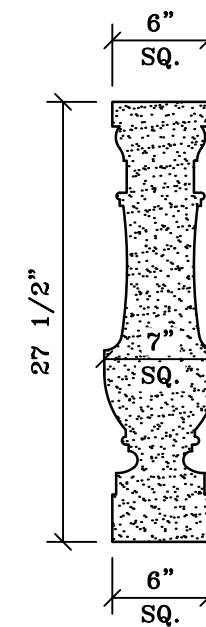
BA-309 Baluster New Baluster
