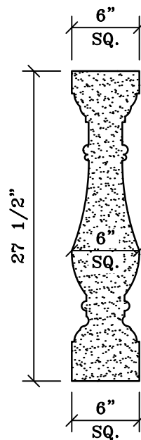
BA-303 Baluster New Baluster
