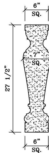
BA-308 Baluster New Baluster
